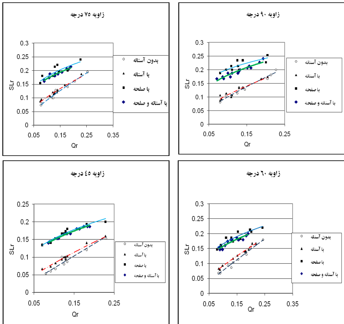
شکل (۱۲) تاثیر آستانه و صفحات مستغرق در عرض جدایی ناحیه گردابی در زوایای مختلف آبیگری
