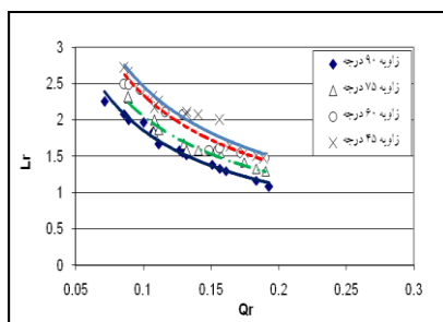
شکل (۵) تغییرات L_r در مقابل Q_r برای زوایای مختلف آبیگری
