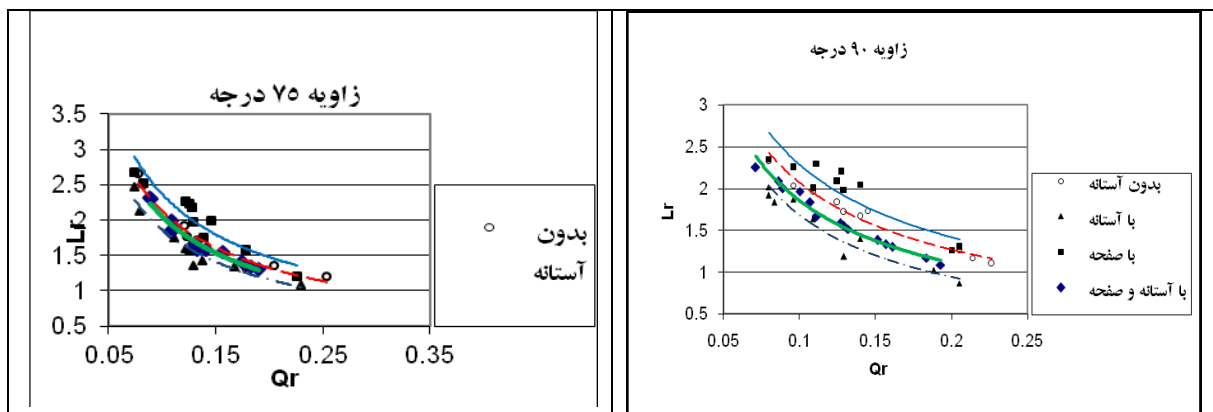
شکل (۷) تأثیر آستانه و صفحات مستغرق در طول نسبی ناحیه گردابی در زوایای مختلف آبیاری
