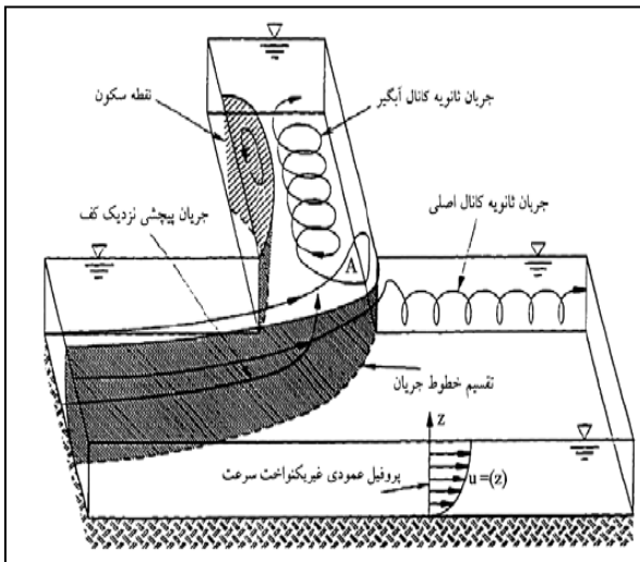
شکل (۱) الگوی جریان ورودی به آبرگیر جانبی
