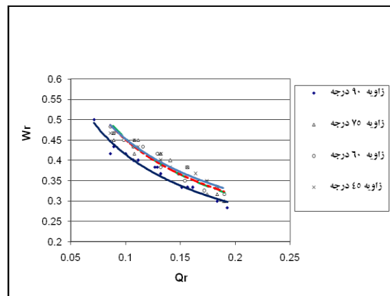
شکل (۸) تغییرات W_r در مقابل Q_r در حالت وجود توأم آستانه و صفحات مستغرق در زوایای مختلف آبیگری
