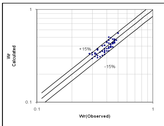
شکل (۹) مقایسه مقادیر W_r مشاهده‌ای و محاسبه‌ای از رابطه
