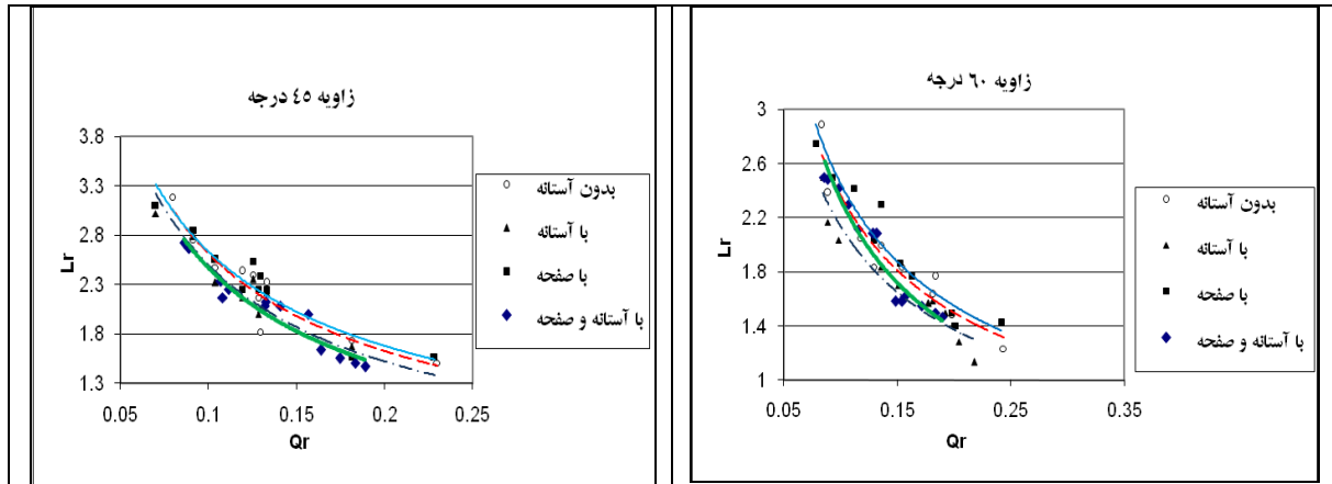
ادامه شکل (۷) تاثیر آستانه و صفحات مستغرق در طول نسبی ناحیه گردابی در زوایای مختلف آبیگری
