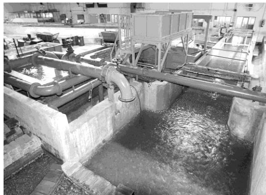
شکل (۳) نمایی از فلوم مورد استفاده در آزمایشات
