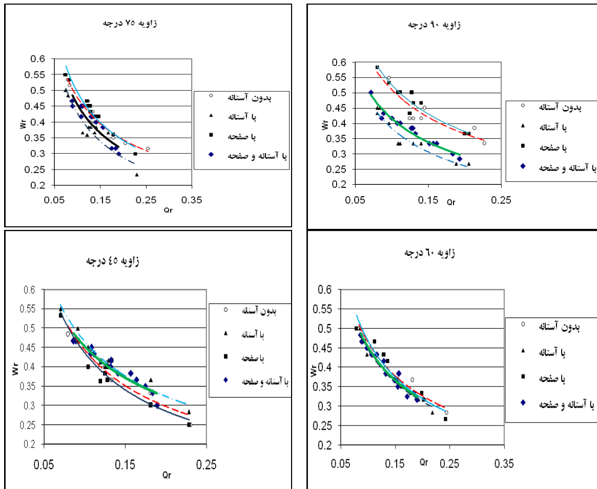
شکل (۱۰) تأثیر آستانه و صفحات مستغرق در عرض نسبی ناحیه گردابی در زوایای مختلف آبگیری
