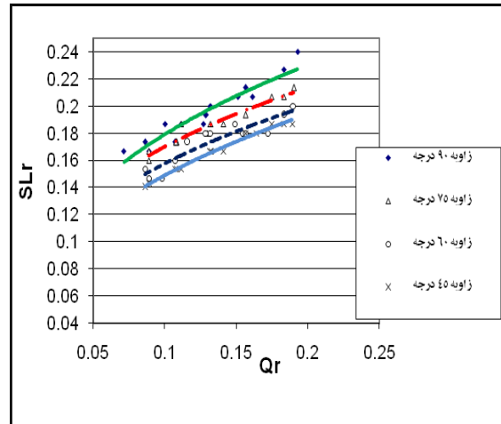
شکل (۱۱) تغییرات SLr در مقابل Qr در حالت وجود توأم صفحه و آستانه برای زوایای مختلف آبیگری
