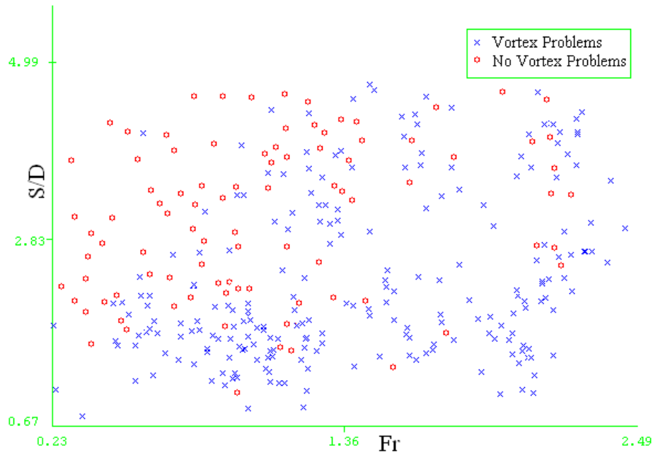
شکل (۵): وضعیت خطر وقوع جریان گردابی در آبگیر قائم به ازای L/w=2.25
