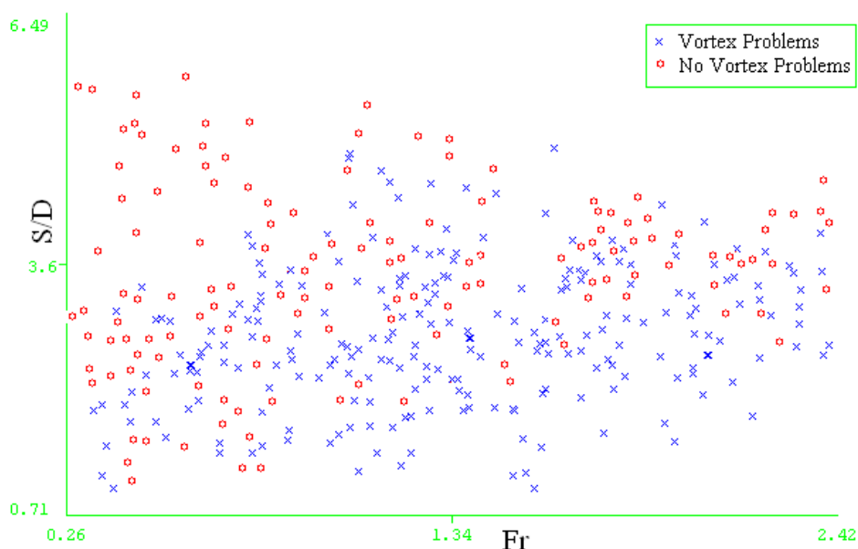
شکل(۴): وضعیت خطر وقوع جریان گردابی در آبگیر قائم به ازای L/w=1.13
