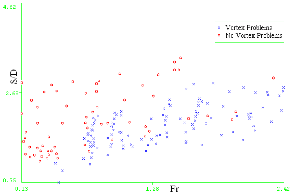
شکل (۶): وضعیت خطر وقوع جریان گردابی در آبگیر قائم به ازای L/w=3.56
