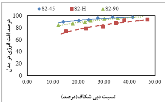
شکل(۸): تغییرات درصد افت انرژی در مدل در برابر درصد دبی شکاف در مدل S۲
