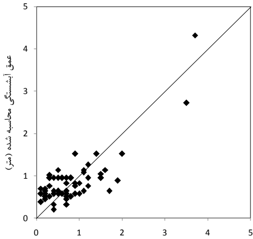
عمق آیشستگی مشاهده‌ای (متر) عمق آیشستگی محاسبه شده (متر) (د) مدل CART- مرحله صحت سنجی
