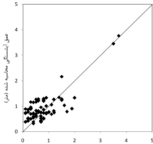
عمق آیشستگی مشاهده‌ای (متر) عمق آیشستگی محاسبه شده (متر) (ب) مدل M5- مرحله صحت سنجی
