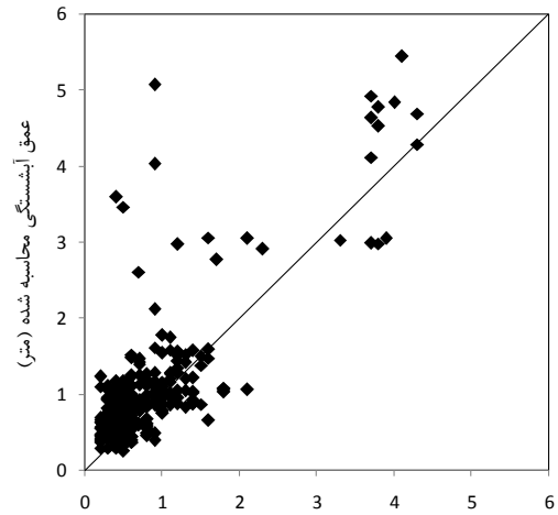
عمق آیشستگی مشاهده‌ای (متر) عمق آیشستگی محاسبه شده (متر) (الف) مدل M5- مرحله آموزش
