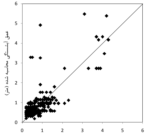
عمق آیشستگی مشاهده‌ای (متر) عمق آیشستگی محاسبه شده (متر) (ج) مدل CART- مرحله آموزش
